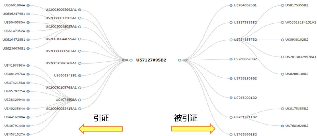
图 2-6 引证关系图
