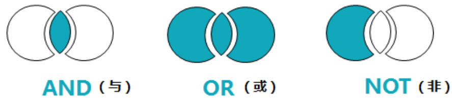
图 2-21 逻辑运算符
